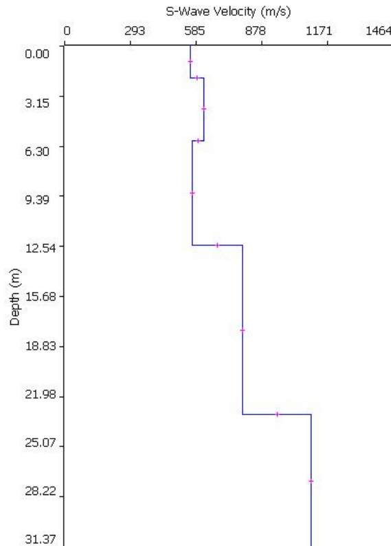
Fig. 8: Distribuzione Vs
