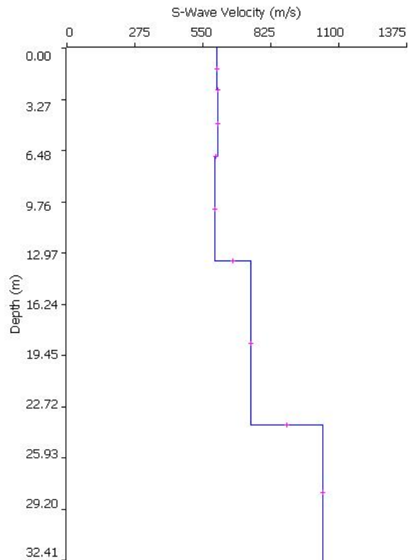
Fig. 12: Distribuzione Vs
