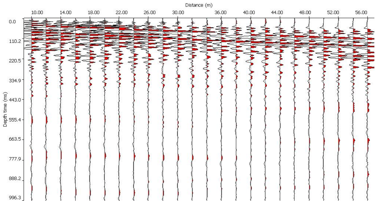
Fig. 9: Sismogramma medio
