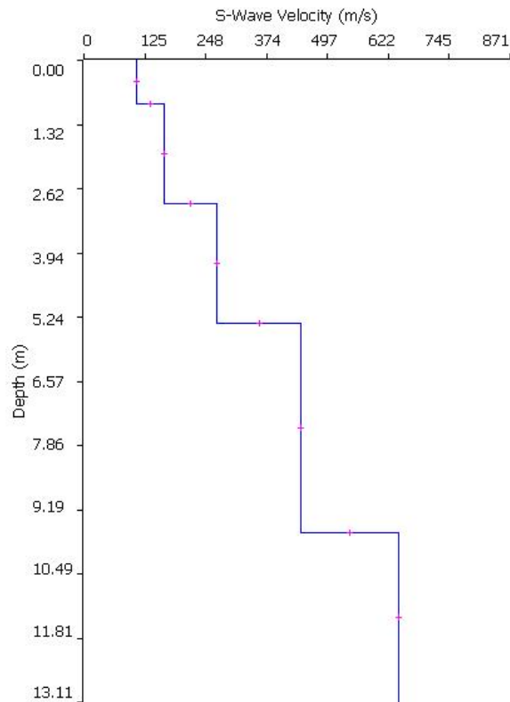
Fig. 16: Distribuzione Vs
