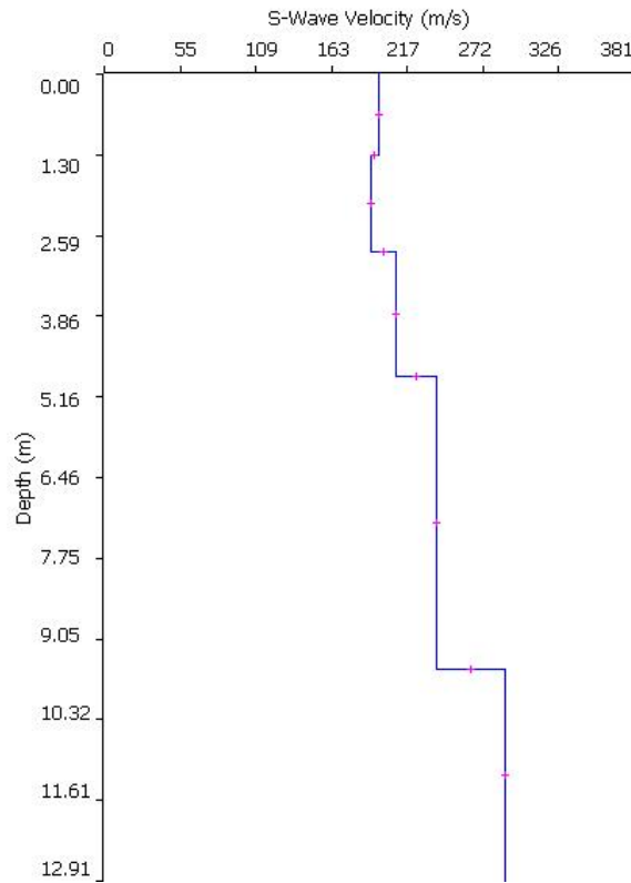
Fig. 4: Distribuzione Vs
