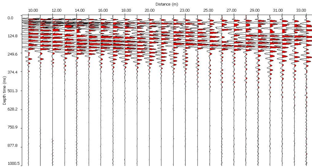
Fig. 25: Sismogramma medio
