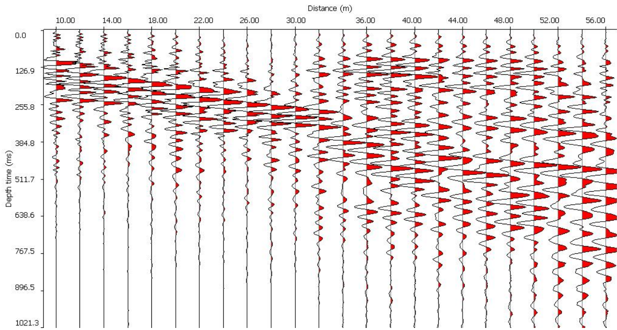
Fig. 17: Sismogramma medio
