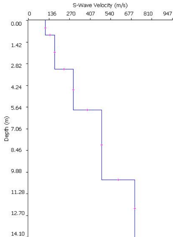
Fig. 20: Distribuzione Vs
