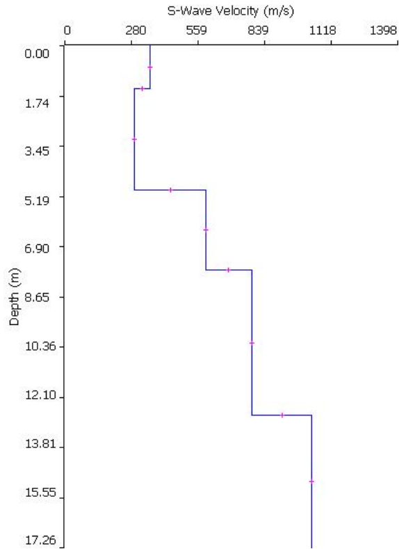
Fig. 28: Distribuzione Vs
